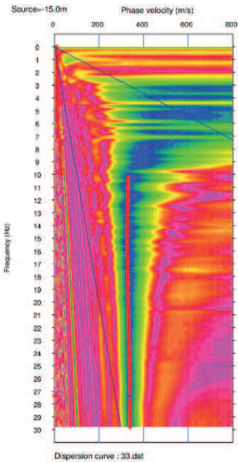
Grafico Velocità di fase-Frequenza (Masw)
